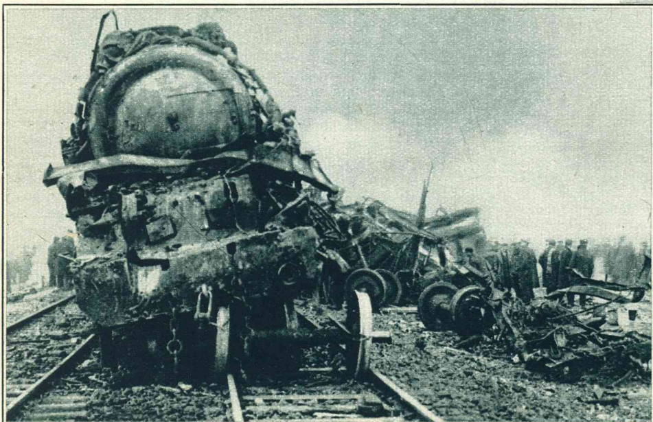
De locomotief van den Straatsburg-expres, die de houten wagons van den ongelukstrein van achteren naar voren totaal uit elkaar sloeg.
