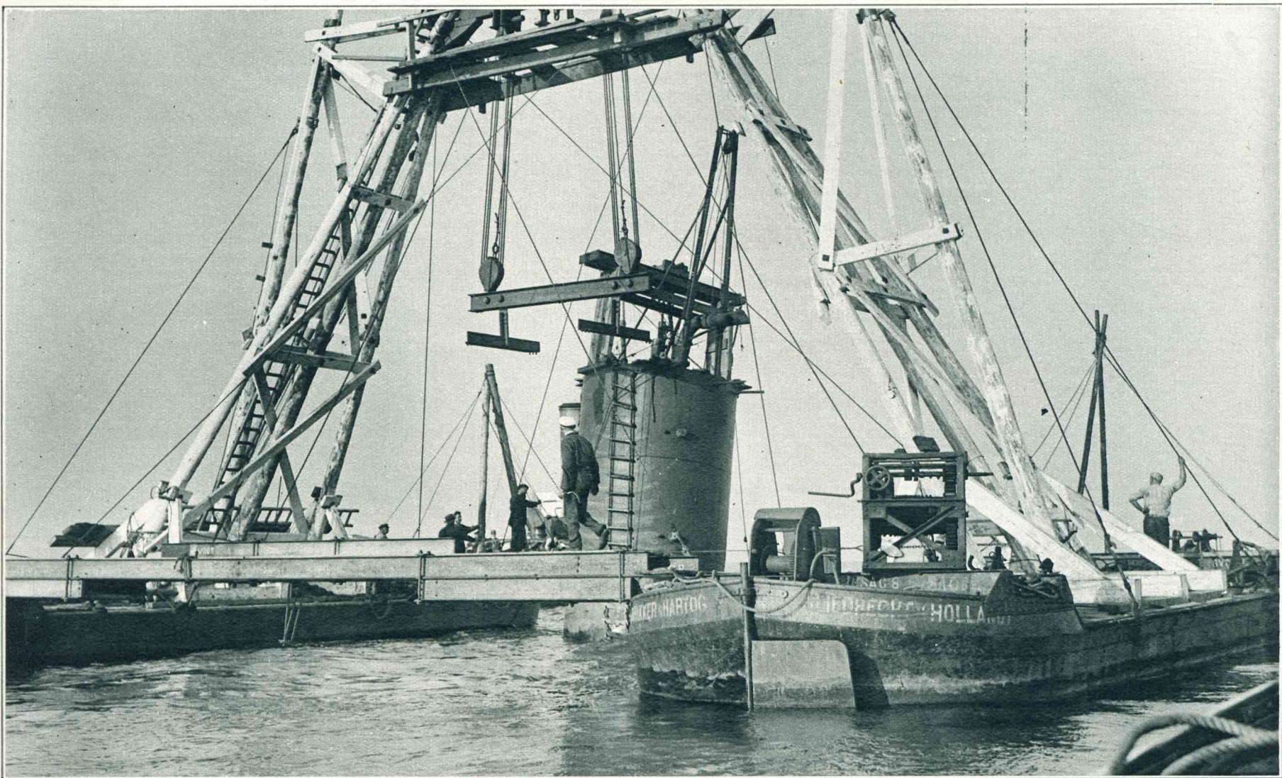
De afbraak boven de Lutine. De bok is boven het wrak gevaren om het cilindervormig gedeelte van den toren te demonteeren, waarna de kegel uit het zand wordt getrokken.
