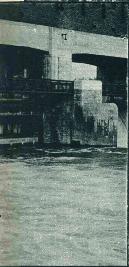
De trap voor de visschen, een langzaam stijgende reeks van treden achter elkaar, waar de visschen van 't eene bassin in 't andere kunnen springen.
