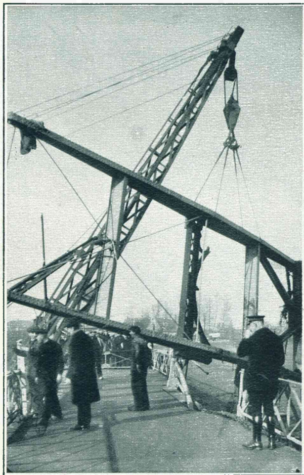
De belemmering opgeheven. Met 'n drijvende bok is het bovenstuk van de brug over de Linge te Geldermalsen, dat onlangs door een auto in het water werd gereden, verwijderd. De scheepvaart, die tot dusver gestremd was, kan daarmede weer doorgang vinden.
