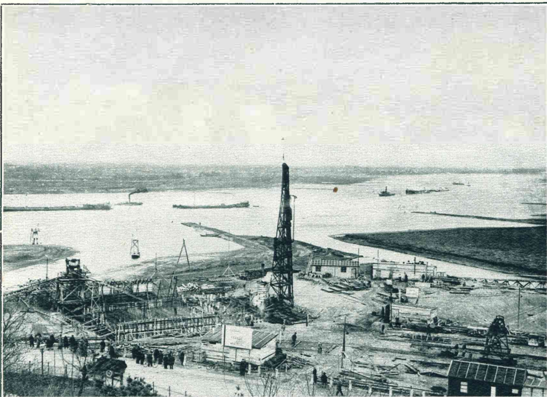
Het begin is er, en dat begin vordert goed. Nu het zware heilwerk voor het landhoofd van de Waalbrug te Nijmegen gereed is, werd begonnen met het storten van het beton. Wij geven op deze foto een overzicht van het groote werk, als een blij vooruitzicht op de niet al te verre toekomst, dat ook hier 't water geen tijdroovende belemmering voor het verkeer meer zal zijn.
