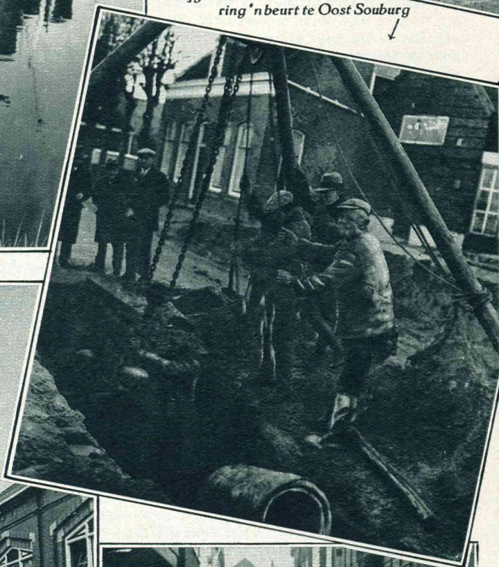
Alvorens de straat definitief wordt gelegd, krijgt eerst de rioleering 'n beurt te Oost Souburg
