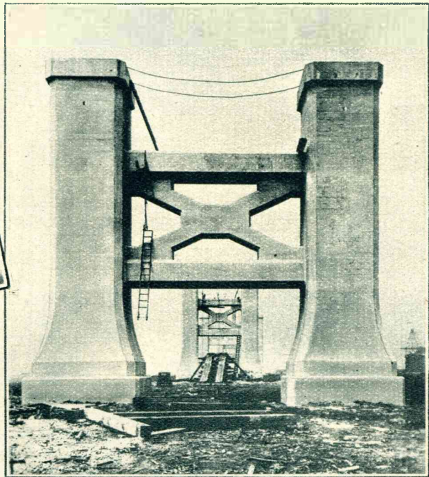
Een der betonnen pijlers van den „hoogen" weg tusschen New Mark en Yersey City, die thans voltooid is.
