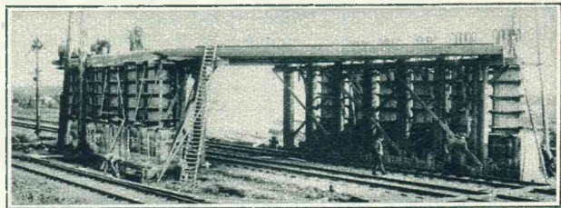
Te 's Heer Arendskerke wordt ten behoeve van 'n nieuwen verkeersweg een viaduct gebouwd over de spoorlijn Roosendaal—Vlissingen: de verkeersweg wordt dus straks over de spoorlijn geleid.
