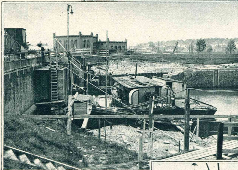
De herstelwerken van een der sluizen te Hansweert nemen een zeer grooten omvang aan, zoodat met het werk heel wat tijd heen gaat. Een overzicht op een deel van het werk.
