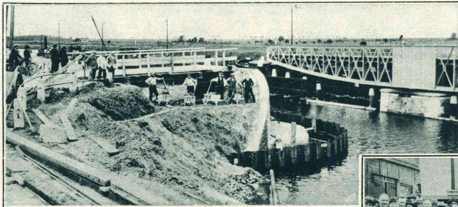
Terwijl men nog bezig is aan het groote sluiswerk te Hansweert, wordt het Kanaal van Zuid-Beveland nog verder verbeterd door bij de Postbrug de doorvaart te verbreden: de bocht wordt er uit weggenomen.
