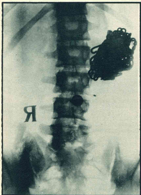
Wat de X-stralen laten zien: een Röntgen-foto van de maag van een mensch, met de ingeslikte voorwerpen, de oorzaak der stoornissen en ziekteverschijnselen.
