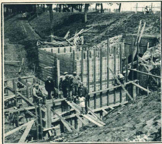
De polder van het waterschap Poortvliet wordt van 'n elektrische bemalingsinrichting voorzien. Een kijkje op het werk.
