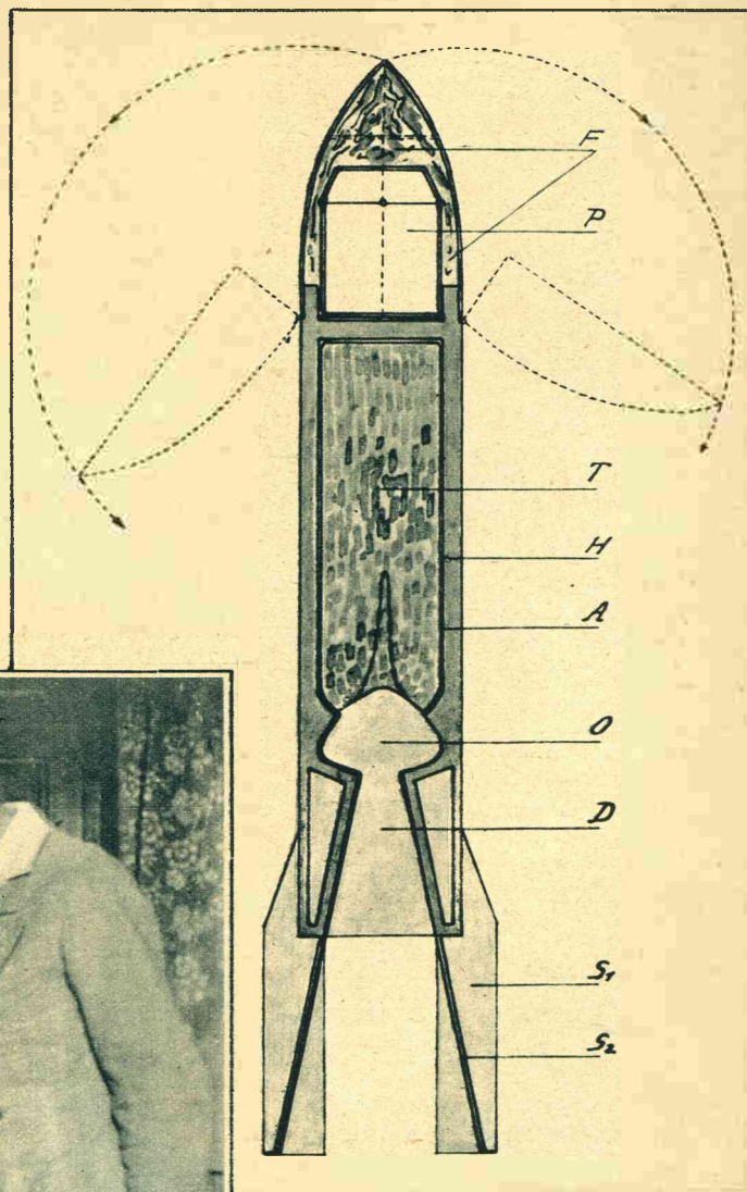
De postraket in doorsnee; F - gevouwen parachute; P - ruimte voor brieven; T - de drijvende kracht; H - rakethuls; A - asbestbekleding; O - stookruimte der gassen; D - uitlaat; S - stabilisatievlakken.
