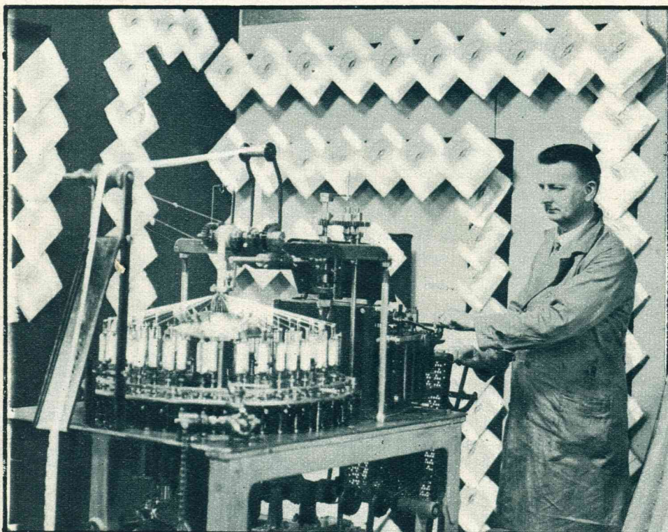
De kantmachine.
