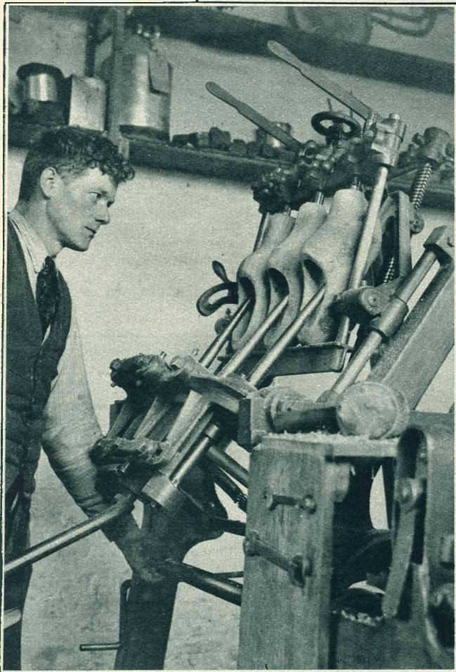
Geleidelijk worden onze Zeeuwsche klompenmakerijen gemoderniseerd en van machines voorzien, waarmee dan de klompen worden gemodelleerd en afgemaakt. Een kijkje in zoo'n gemoderniseerde klompenmakerij te Goes.
