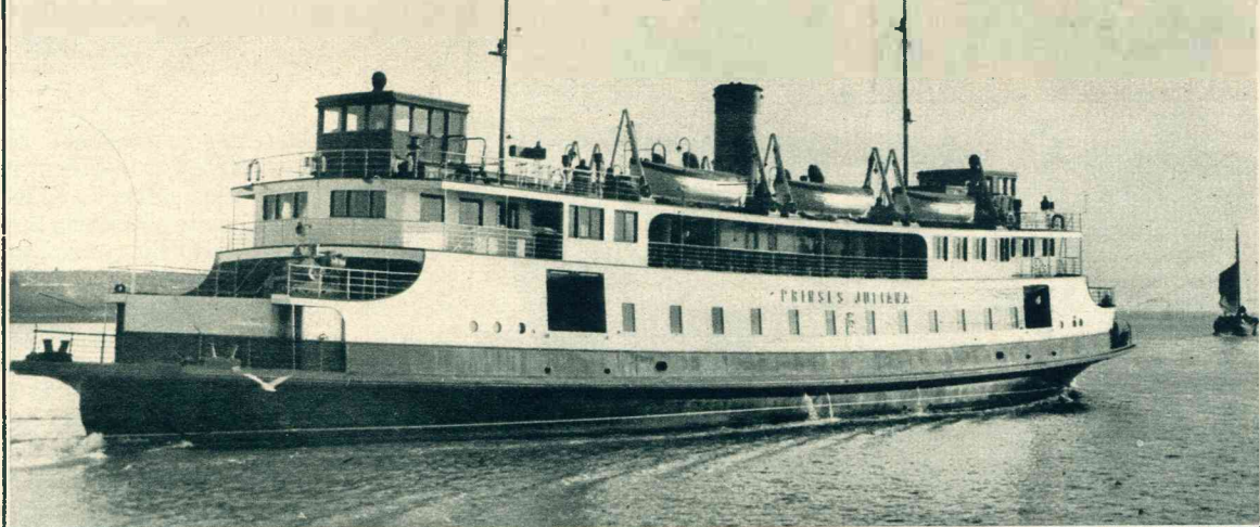
Foto van het nieuwe schip in de vaart. Er kunnen ruim 5000 passagiers en 50 à 60 auto's mee overgezet worden.
