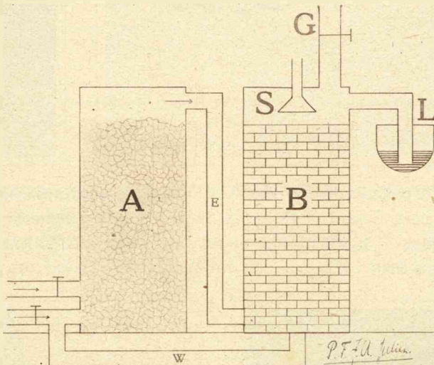
Schematische voorstelling van een watergasfabriek. Verklaring in den tekst.
