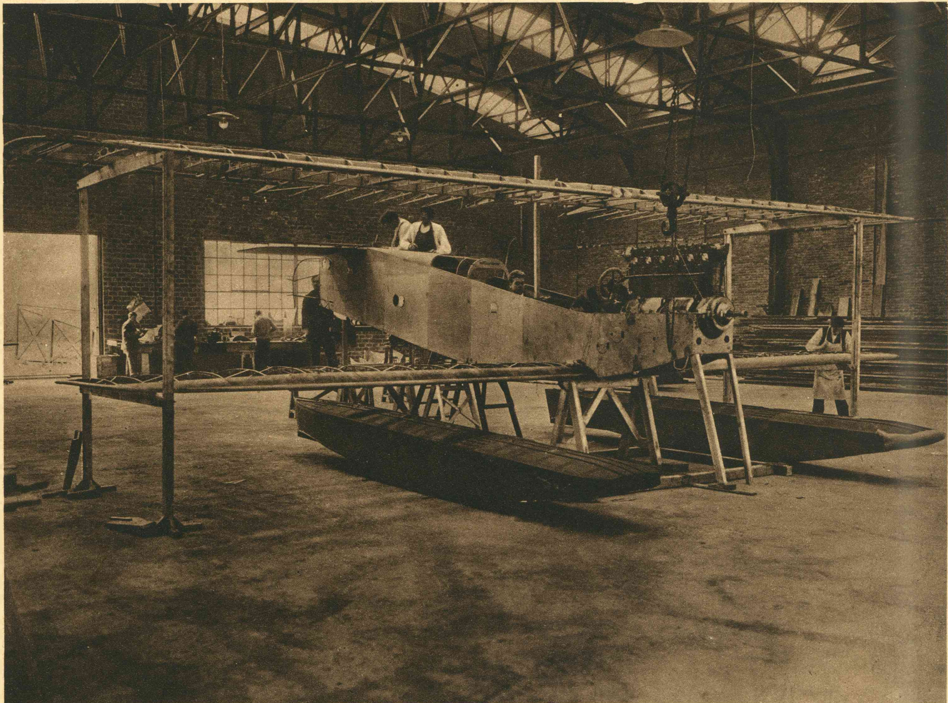
Het vliegtuig in de montage-afdeeling.
