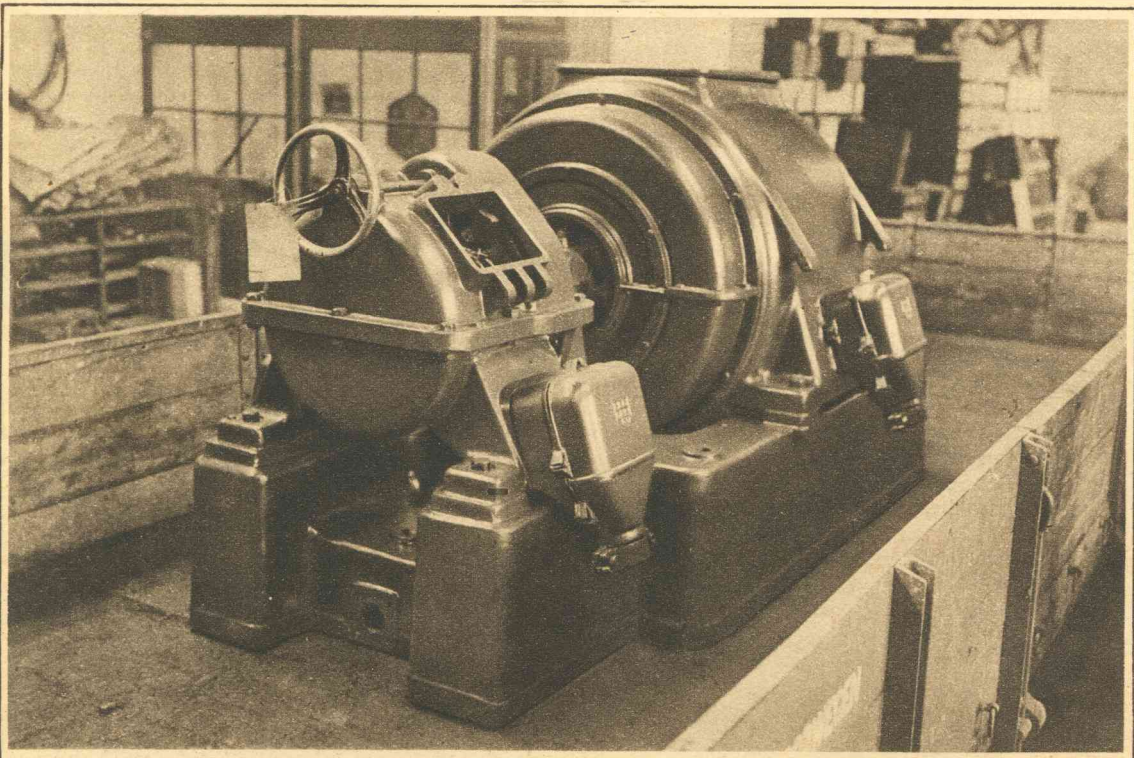
TURBOMOTOR VOOR MIJNBEDRIJF (1500 TOEREN, 750 P.K.)
