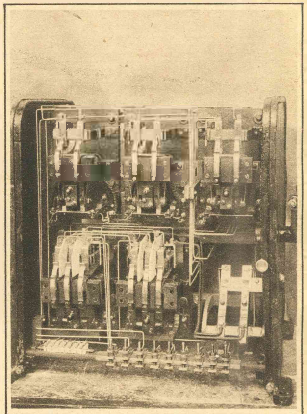
Liftschakelaar.
