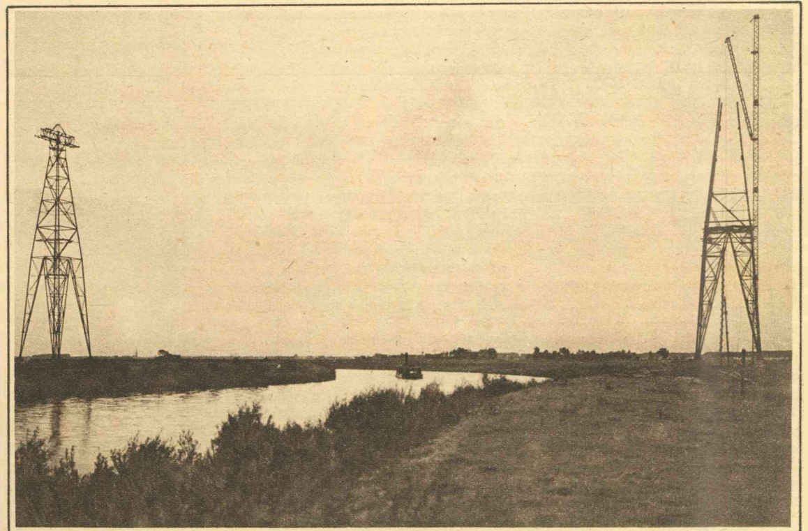
KABELMASTEN. — RIVIERKRUISING VAN 50.000 VOLT LIJN.
