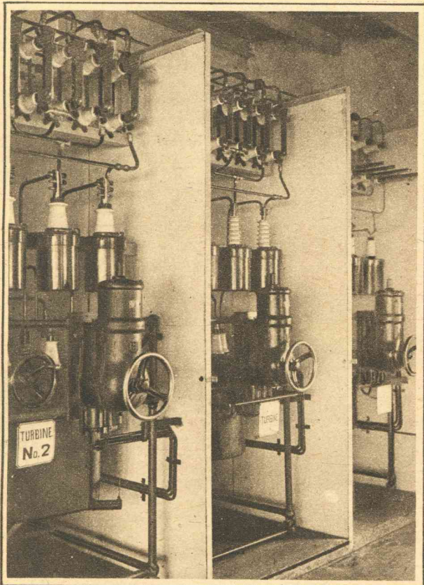
Schakelcellen, 10.000 volt, aanleg.
