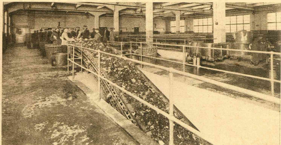
NIEUWE GEMEENTELIJKE VUILVERBRANDING TE AMSTERDAM. Een kijkje in de sorteerinrichting van de nieuwe gemeentelijke inrichting voor vuilverbranding te Amsterdam aan den Overkant van het IJ. Het vuil wordt op een breede transportbaan g worpen en jongens halen de voden, het papier enz. eruit.
