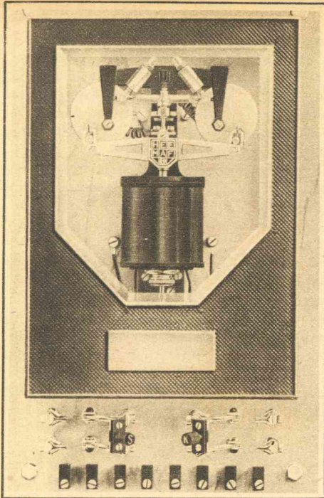
AUTOMATISCHE SPANNINGS-REGELAAR (NEDERL. OCTR. NO. 2293.) Dient om de spanning in centrales bij iedere belasting constant te houden en regelt beter en vlugger dan uit de hand mogelijk zou zijn. (Grootte onderzijde plm. 5 c.M.)
