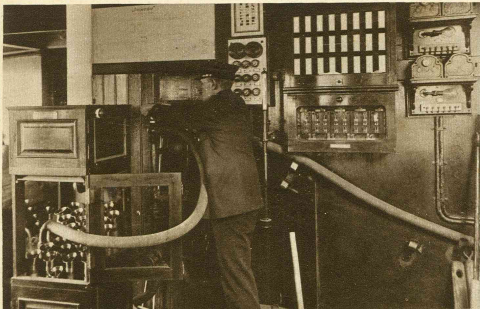
De brandwerktuigen op de commandobrug.
